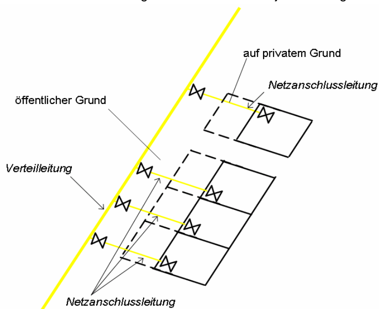
Schema Netzanschluss
